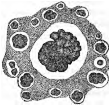
FIG. 47.—ASCOCOCCUS BILLROTHII, X 65. [After Cohn.]
